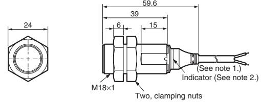
E2A3-M18KS11-WP-□□
